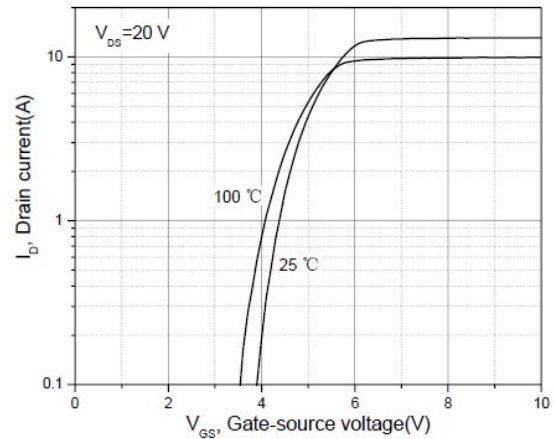
图 4 传输特性曲线
