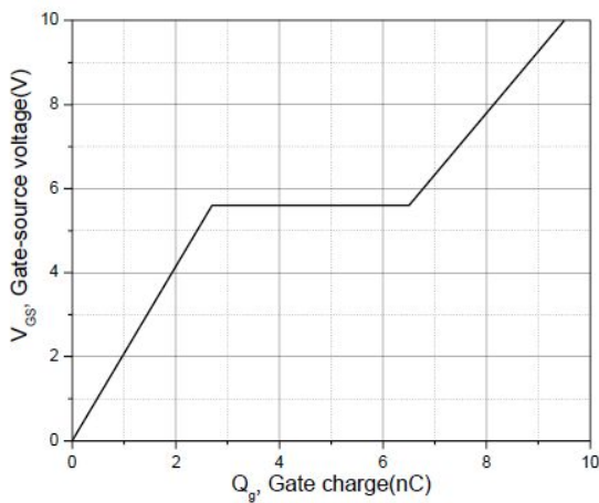
图 9 栅电荷与 VGS 关系曲线 Fig9 Gate Charge waveforms
