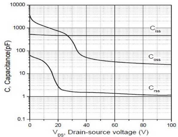
图 10 电容与漏源电压关系曲线 Fig10 Capacitance
