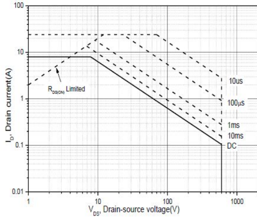
图 1 最大安全工作区曲线
