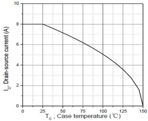
图 8 最大 ID 与结温曲线 Fig8 Maximum ID VS Junction Temperature
