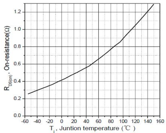
图 6 导通电阻与结温曲线
