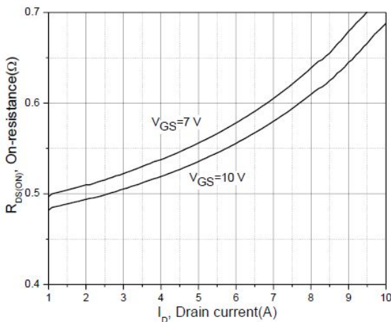
图 5 静态导通电阻与电流曲线
