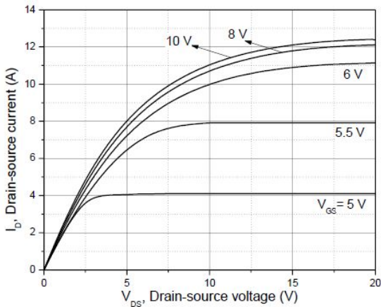
图 3 输出特性曲线, Tc=25°C
