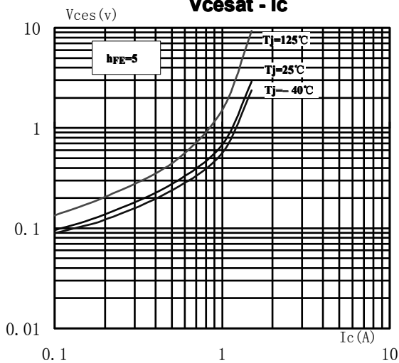
V_{cesat} - I_c
