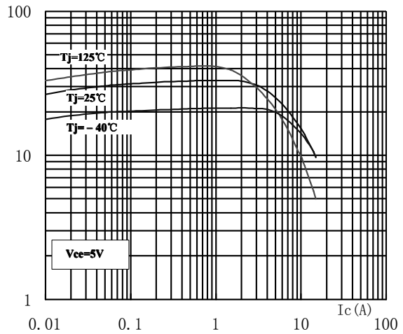
h_{FE} - I_c
