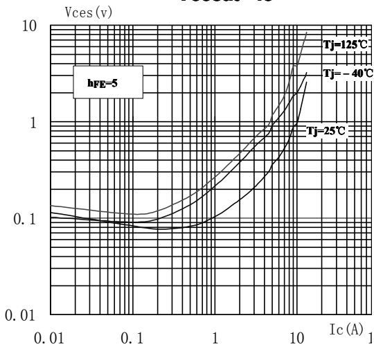
V_{cesat} - I_c
