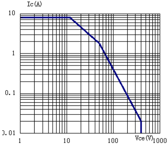
SOA (DC)
